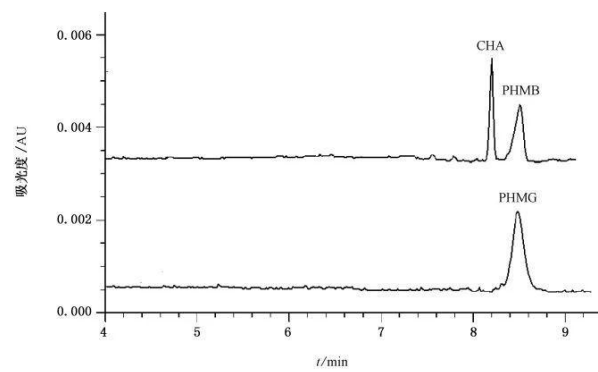
图 B.1 PHMB、PHMG、CHA 的毛细管电泳图
